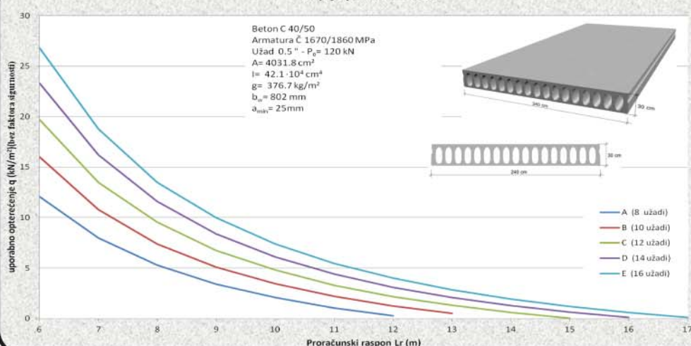
Šuplja ploča h= 30cm
