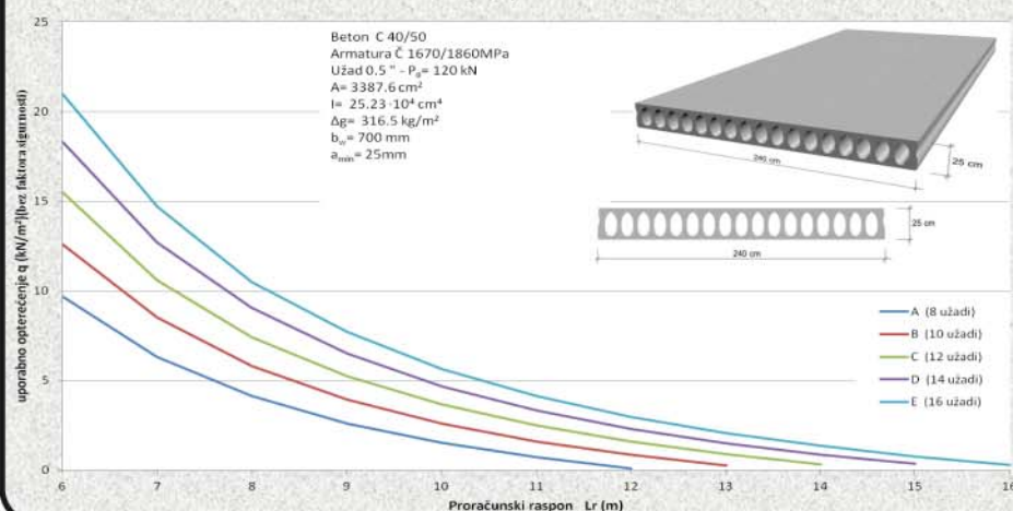
Šuplja ploča h= 25cm
